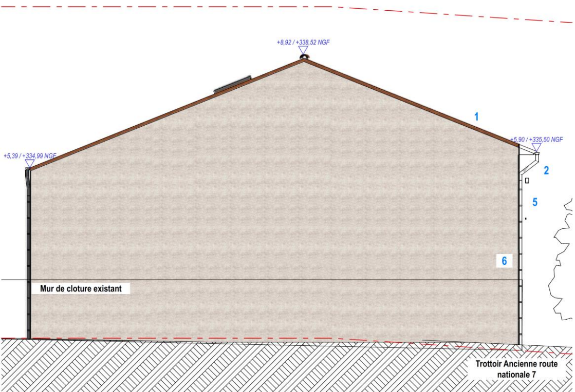
Façade Nord
