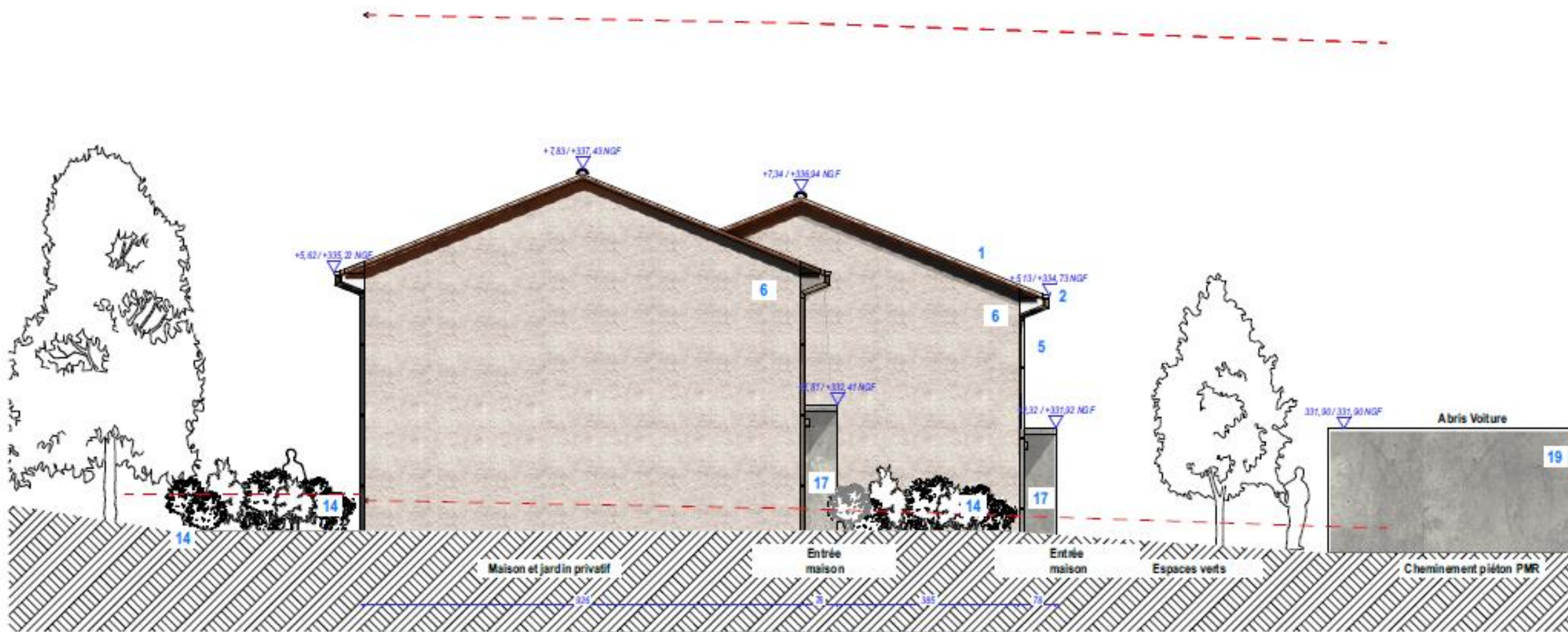
Façade Nord
